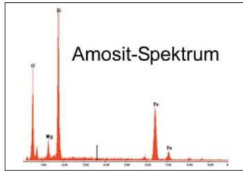
Abb. 5: REM-Identifikationsspektrum von Amosit
