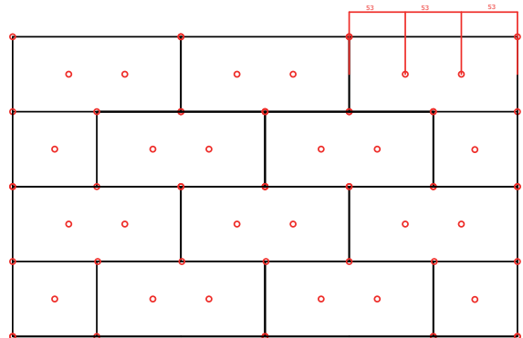
Dübelschema zur nachträglichen Befestigung
