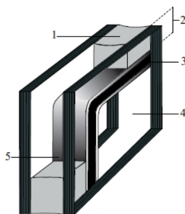
Abbildung 1: Typischer Schnitt Einer Zweifach Abgedichteten Isolierglaseinheit.
