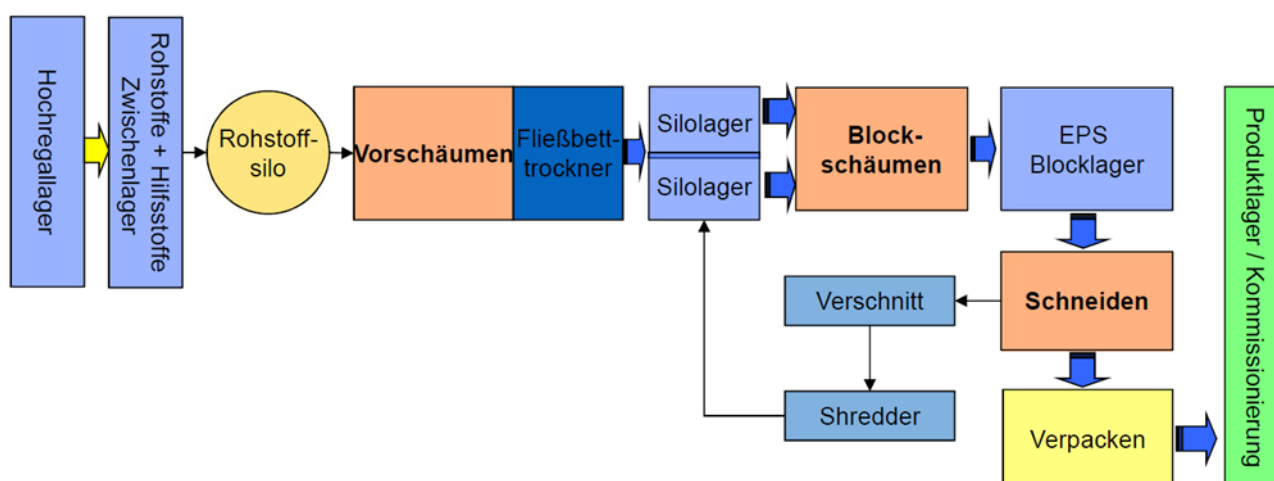
Abbildung 1: Flussdiagramm Herstellungsprozess
