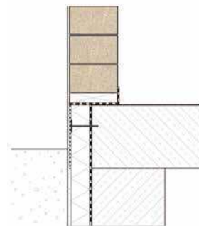
Anschluss gedämmter Keller
