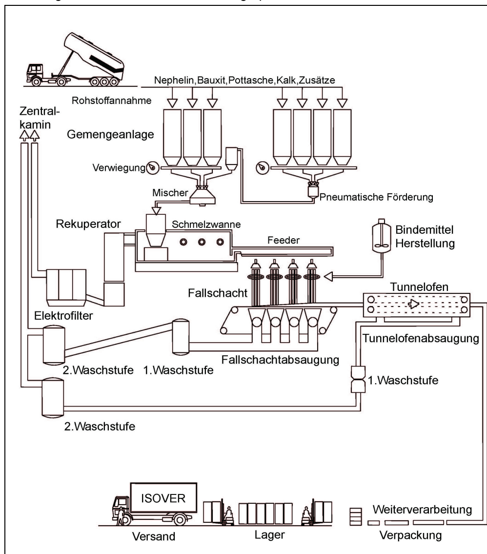
Abbildung 1: Prozessablauf ULTIMATE
