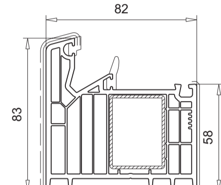
101.291 Verstärkung 113.001, 113.367
