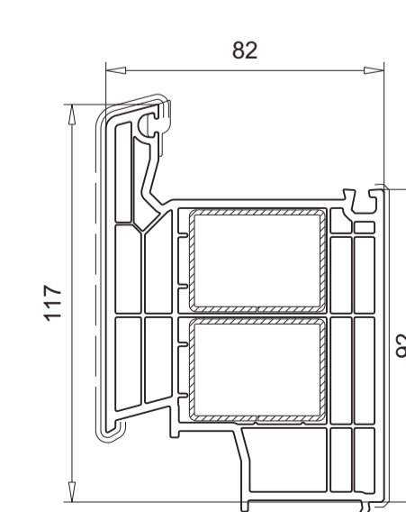
105.382 Aufbauprofil Verstärkung 113.001, 113.001.3
