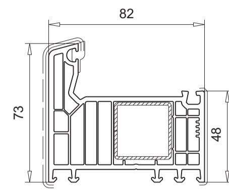
101.293 Verstärkung 113.025, 113.365
