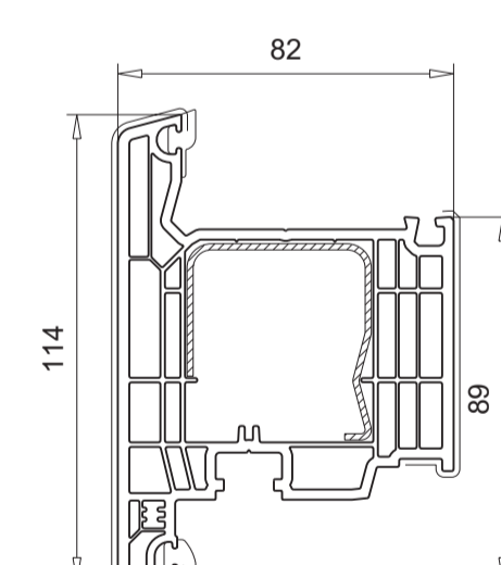
103.346 außen öffnend Verstärkung 113.270, 113.368.2, 115.003
