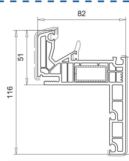
111.052* Verstärkung 113.055
