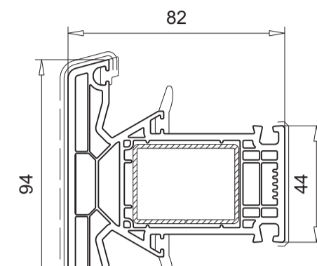
102.310 Verstärkung 113.001, 113.001.3, 113.367
