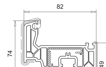
103.340 Verstärkung 113.363
