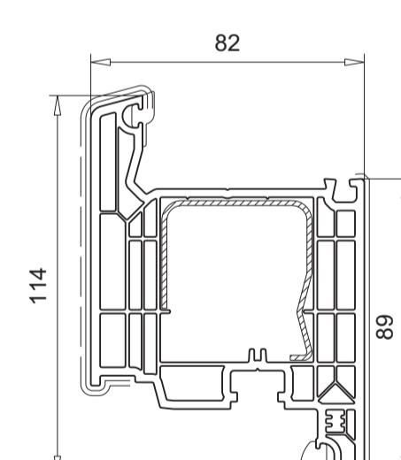
103.345 Verstärkung 113.270, 113.368.2, 115.003
