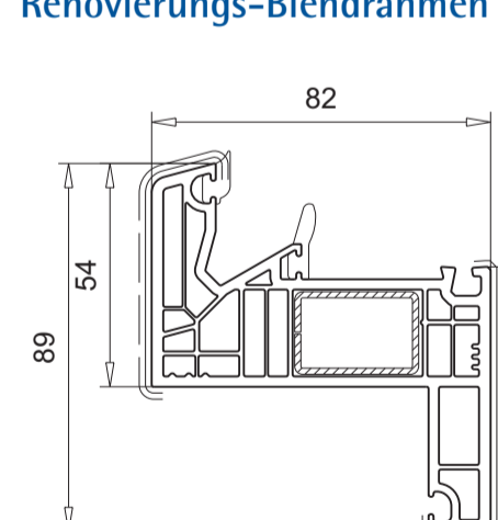
101.300 Verstärkung 113.019
