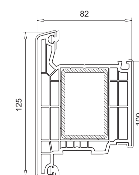
105.381 außen öffnend Verstärkung 113.011.3, 113.011.5 vorgefräst
