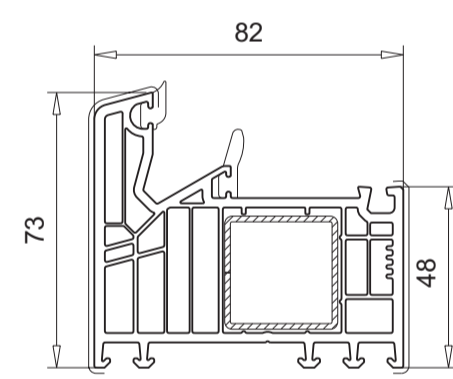
101.295* Verstärkung 113.025, 113.365
