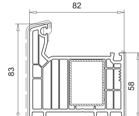
101.294 Verstärkung 113.001, 113.367
