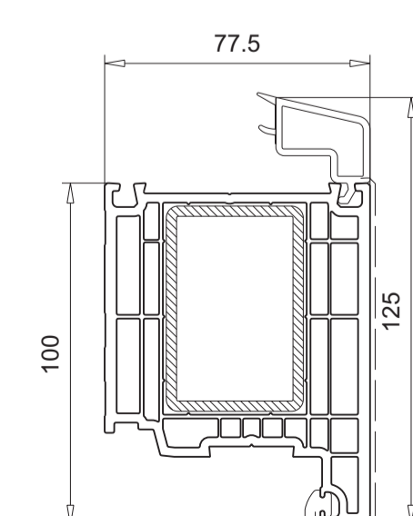
105.383* für flügelüberdeckende Füllungen Verstärkung 113.011.3, 113.011.5 vorgefräst
