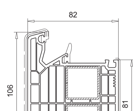
101.292 Verstärkung 113.025, 113.365
