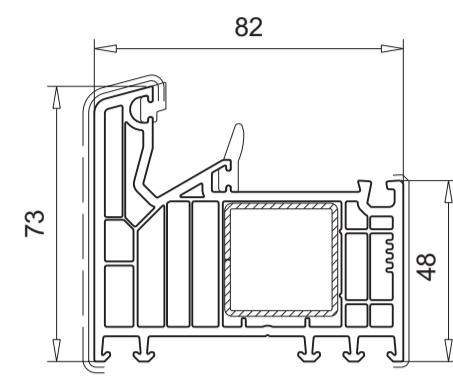
101.290 Verstärkung 113.025, 113.365
