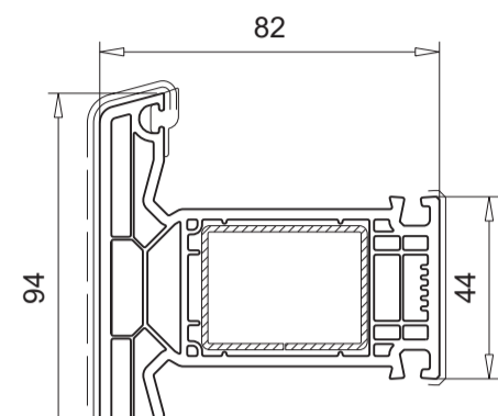
102.312 Verstärkung 113.001, 113.001.3, 113.367
