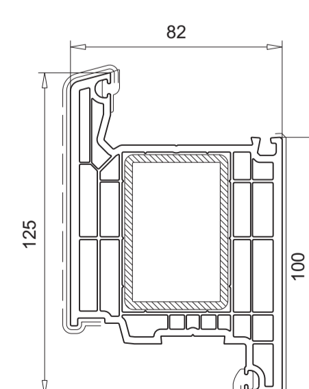
105.380 Verstärkung 113.011.3, 113.011.5 vorgefräst
