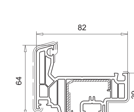
103.358* passend zu 103.341 Verstärkung 113.292, 113.294.2
