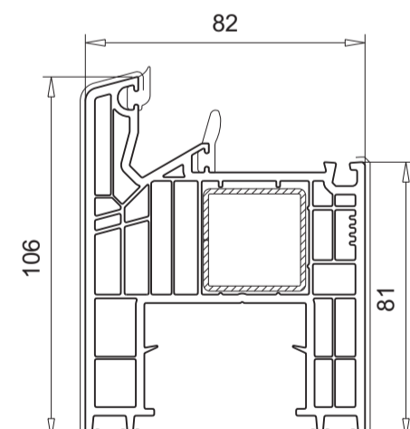
101.296* Verstärkung 113.025, 113.365
