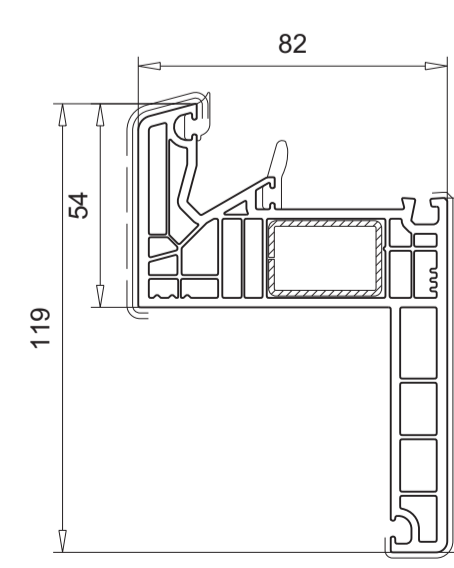
101.301 Verstärkung 113.019
