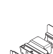
Endkappe zweiteilig 109.664.3 Innenteil Farbe: weiß, schwarz, caramel 109.664.2 Außenteil Farbe: weiß, schwarz, caramel, silbergrau, tannengrün
