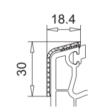
104.277 inkl. Klebeband
