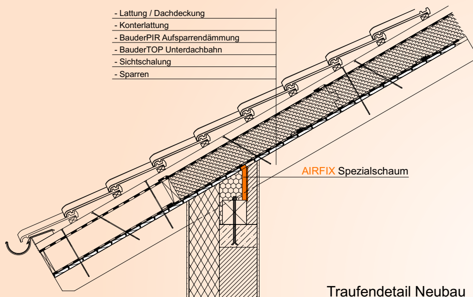
Einbaudetail 2:
