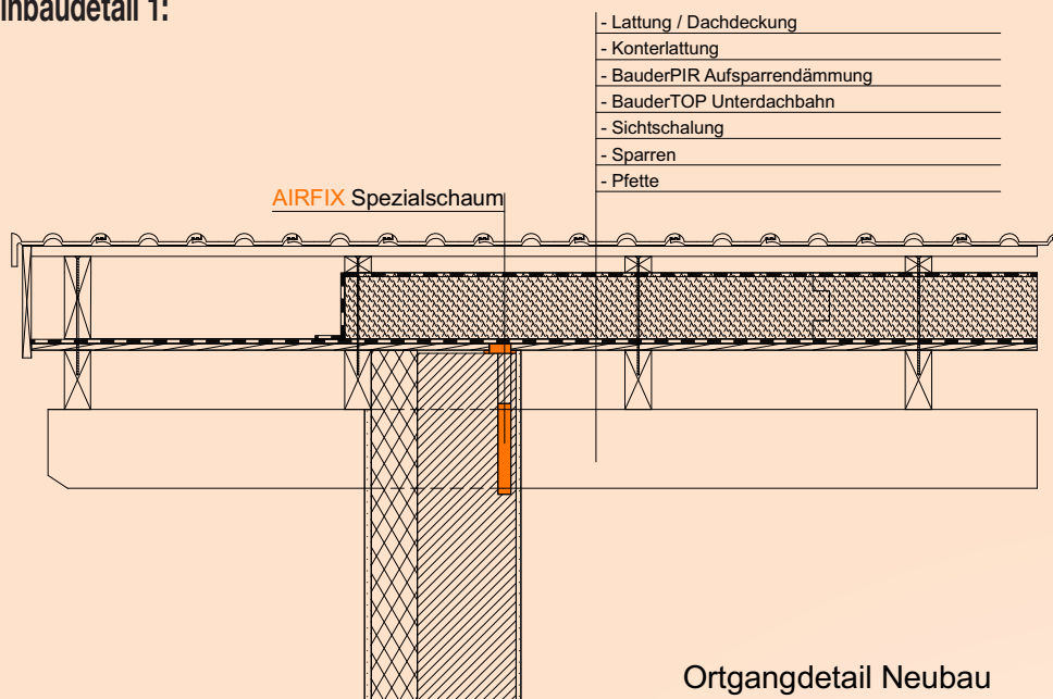
Einbaudetail 1:
