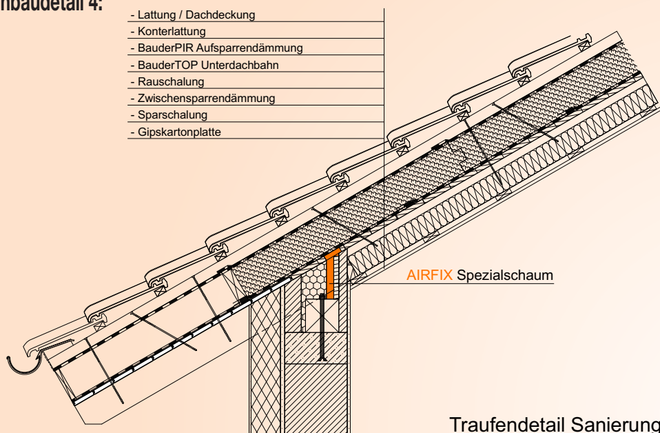
Einbaudetail 4:
