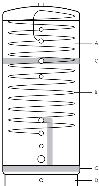
Bild 2: Bauteile des Frischwassermoduls HS-FM035-18
