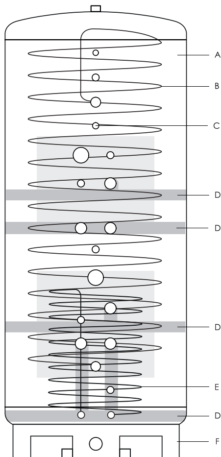
Bild 3: Hauptbauteile der Modelle HS-BM
