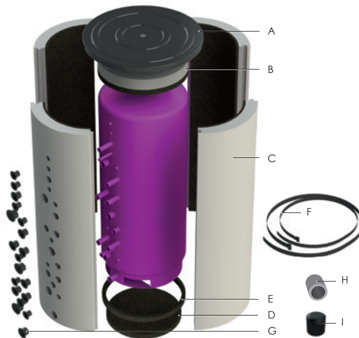
Bild 2: Komponenten Dämmung
