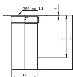
Wavin SX400 Teleskopabdeckung › inkl. Teleskopmanschette, Gussabdeckung B 125 und Kunststoffauflagering* (optional)
